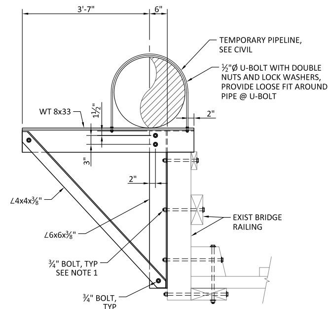
SECTION SCALE: 3/4" = 1'-0"
