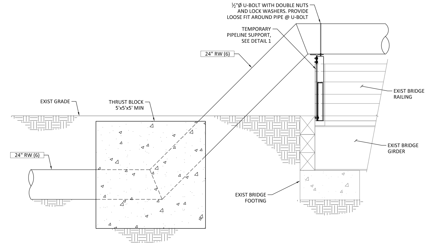
DETAIL SCALE: 1/2" = 1'-0"
